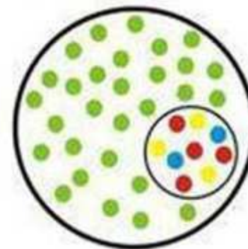
INTEGRARE
