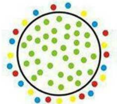
EXCLUZIUNE
