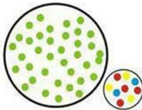
SEGREGARE
