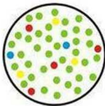
INCLUZIUNE
